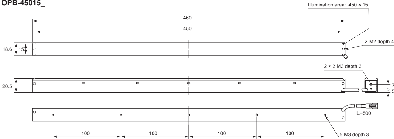
7 OPB-45015_
