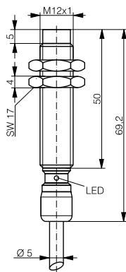
DW-LD-71x-M12
