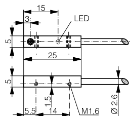
DW-AD-60#-C5
