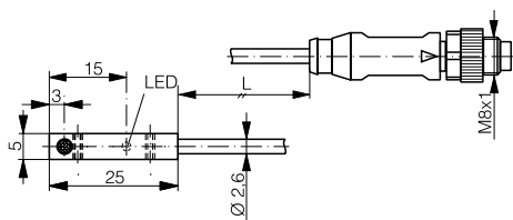
DW-AV-60#-C5-276
